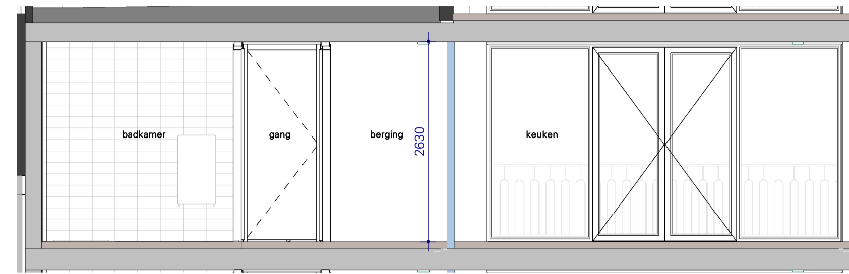
VK Doorsnede A - Blok E -bnr092
